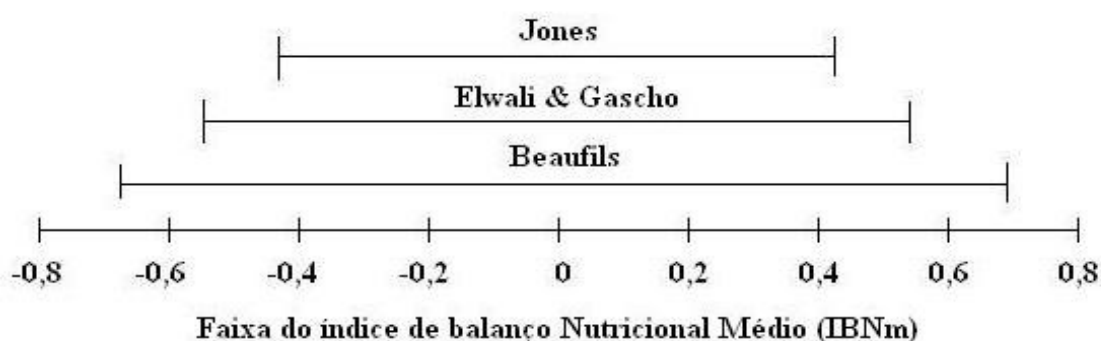
Figura 4 – Representação esquemática do intervalo de suficiência definido pelo IBNm em função de diferentes fórmulas DRIS.
