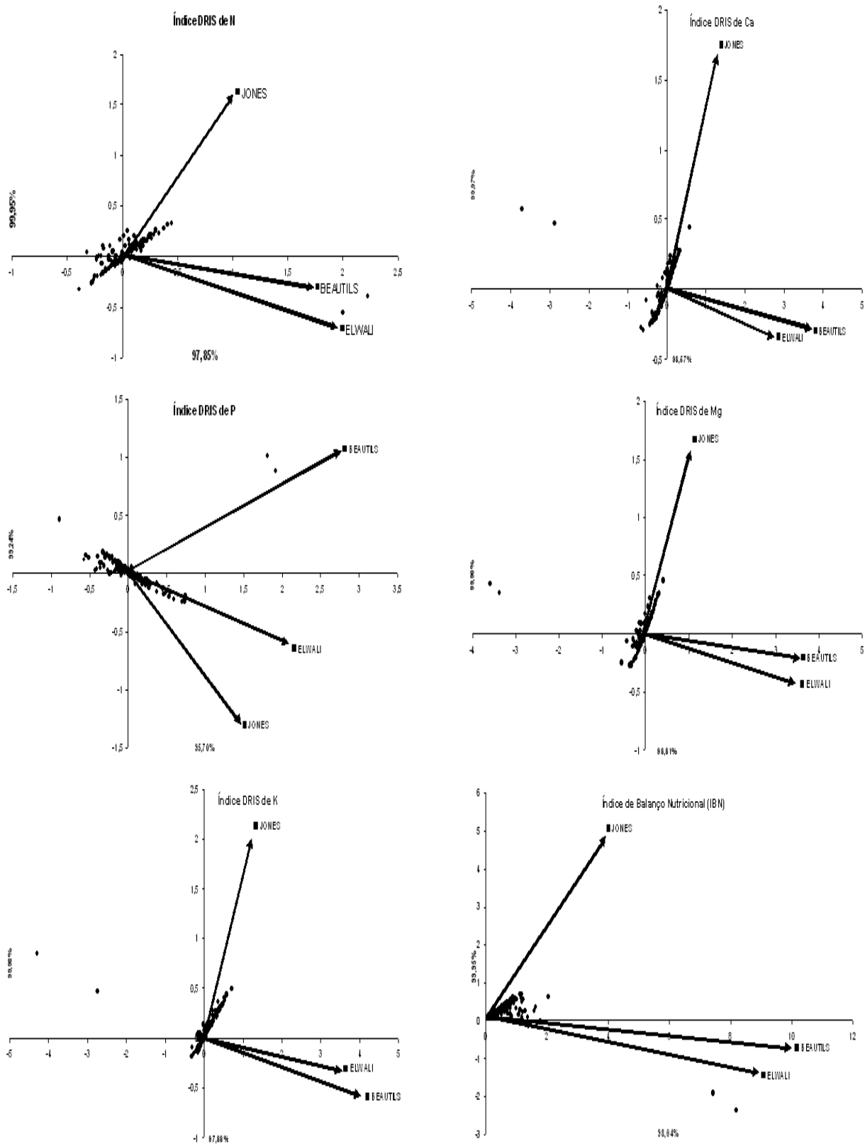
Figura 3 – Distribuição espacial dos índices DRIS proporcionado pela avaliação do estado nutricional de 153 pomares de cupuaçu por diferentes funções DRIS (Beaufils, 1973; Jones, 1981; Elwali; Gascho, 1984).
